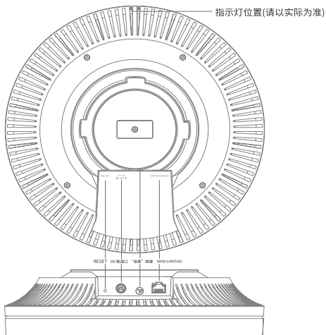
图1-2 底面和侧面示意图
